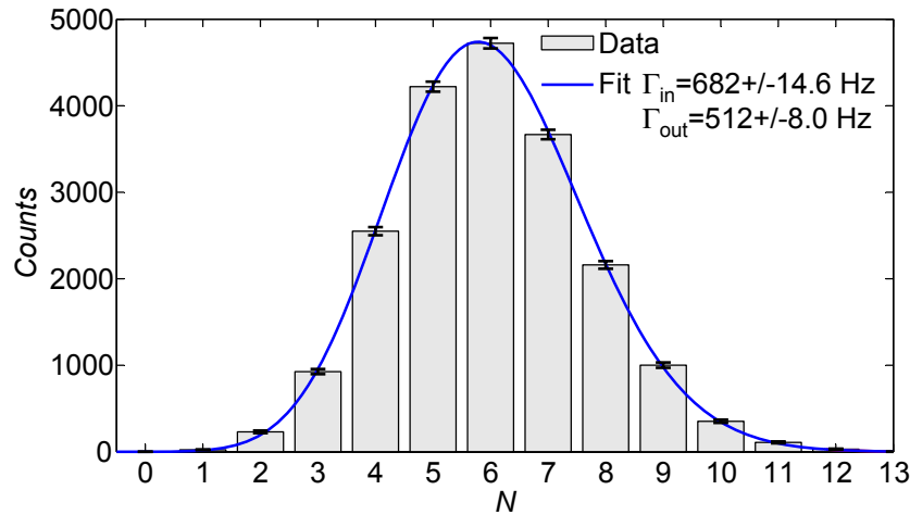
Abbildung 1: Häufigkeit (Counts) einer bestimmten Anzahl N von Ereignissen innerhalb eines Messintervalls. Die durchgezogene Linie ist ein Fit, der nach der Methode der kleinsten Fehlerquadrate durchgeführt wurde.
